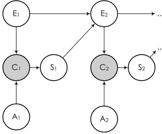
Рис. 3: Модель DBN: байесовская сеть
