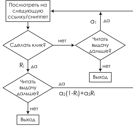
Рис. 1: Модель CSM: блок-схема
